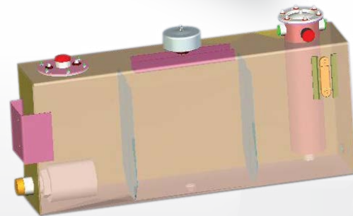
改进后 150加仑液压油箱
