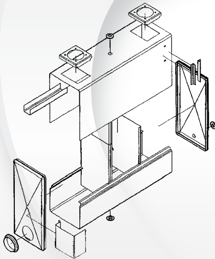
改进前 150加仑液压油箱
